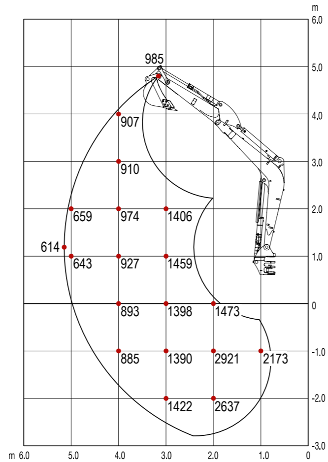
NACH VORN, PLANIERSCHILD ANGEHOSEN
